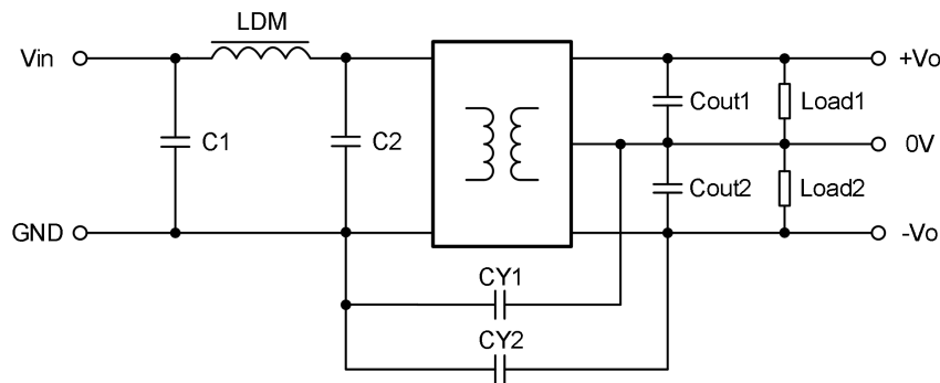
图 2 EMC 推荐电路图
