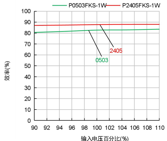
效率与输入电压关系曲线图(满载)
