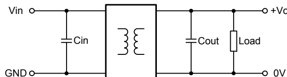
图 1 应用电路图
