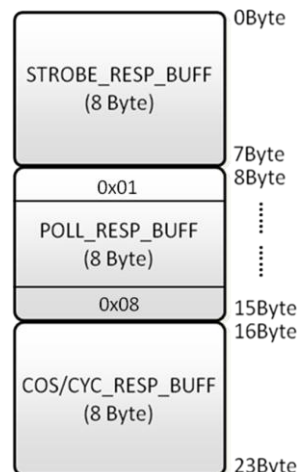
图 5.1 向轮询应答区写入输出数据
