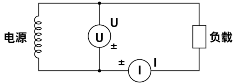
U-I 接线
