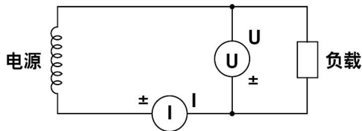
I-U 接线
