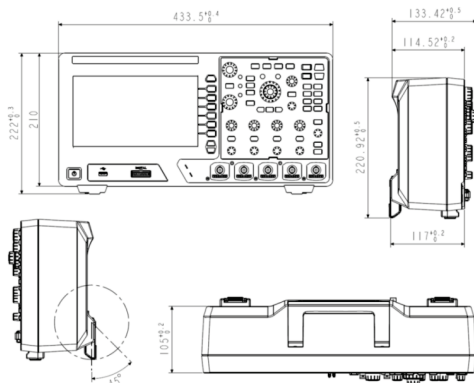
图 4.1 ZDS2000C 示波器尺寸图
