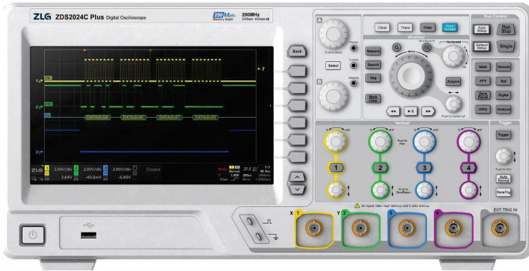
图 3.1 ZDS2024C Plus 示波器面板
