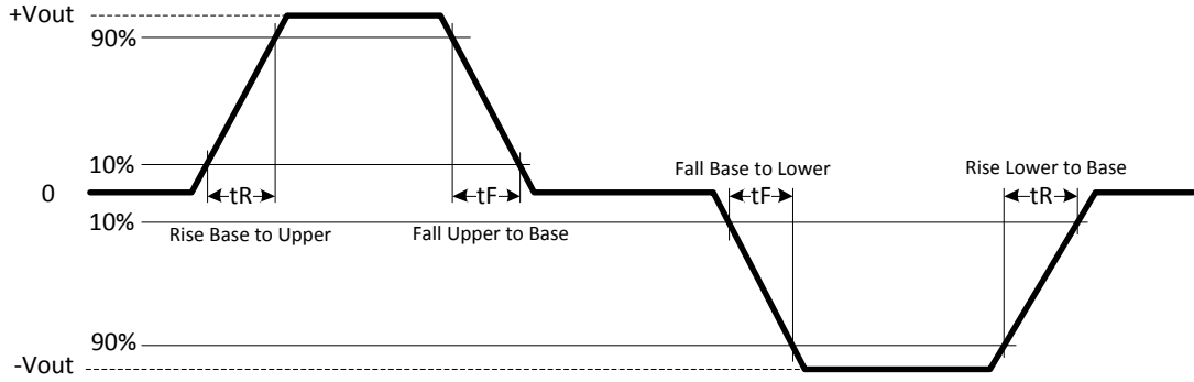
图 3.3 上升和下降时间测试定义
