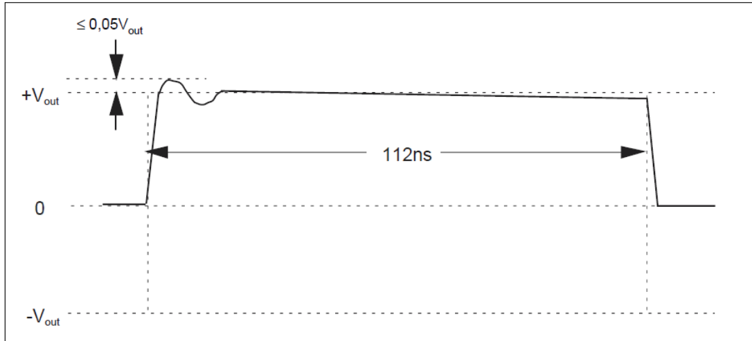
图 3.2 正向过冲
