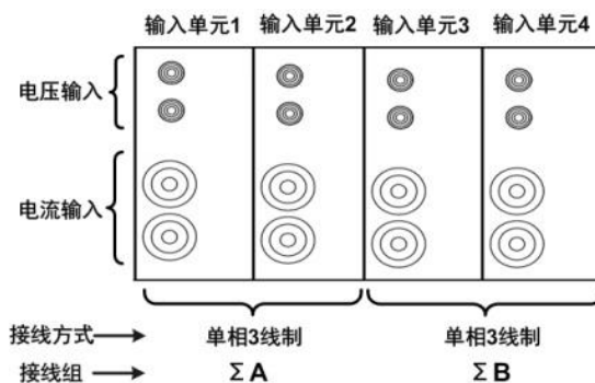
图 2.20 接线组
