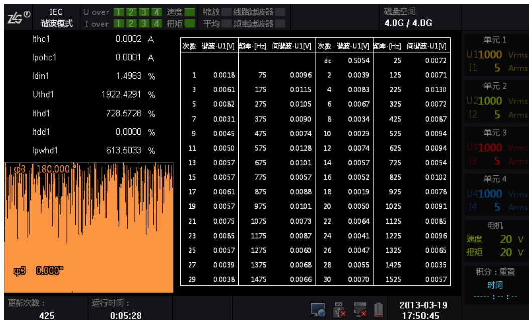
图 2.11 IEC 谐波测量所有视图
