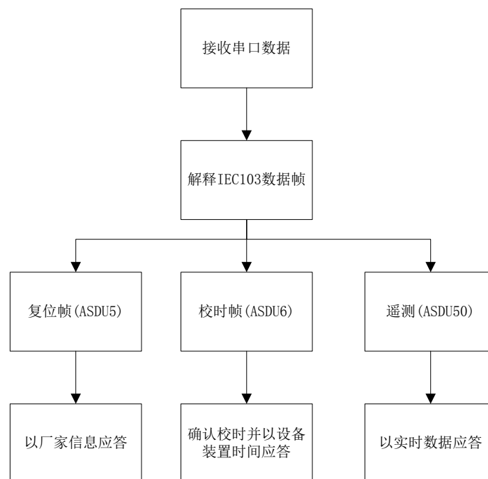
图 3.1 E2000 设备 IEC103 通信基本流程
